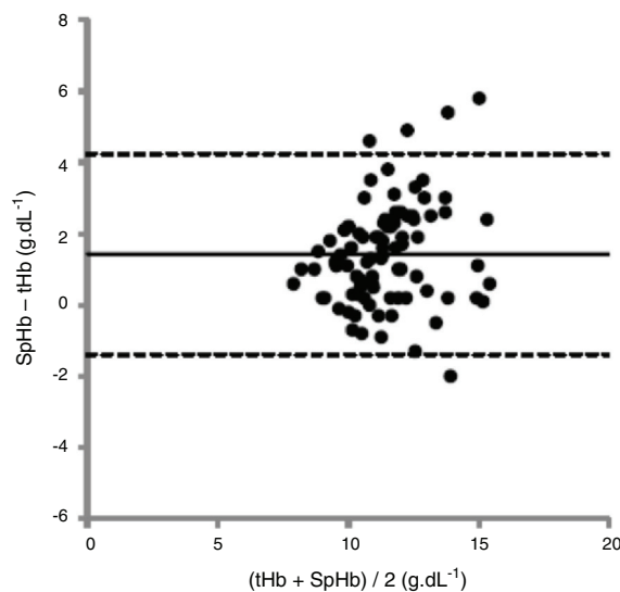
Figura 1 Gráfico de Bland-Altman para a relação geral dos dados entre as diferenças observadas na hemoglobina medida com o CO-Oxímetro de laboratório (tHb) e a monitoração contínua e não invasiva da hemoglobina (SpHb) e a média das duas mensurações.
